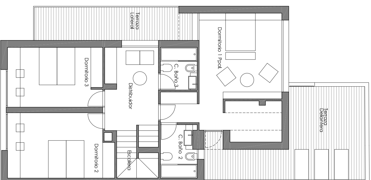
PLANTA PRIMERA
