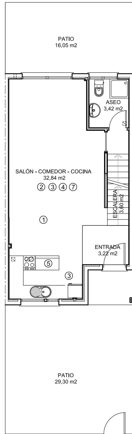
PLANTA BAJA
